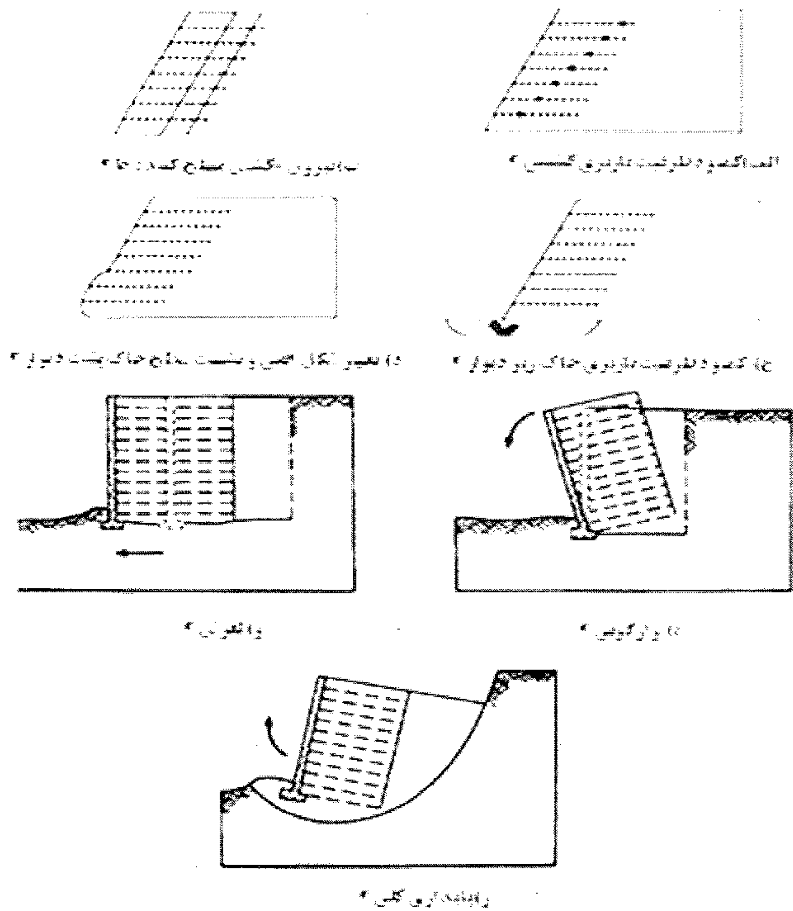
شکل ۷-۵-۲ حالت‌های حدی دیوارهای خاک مسلح
